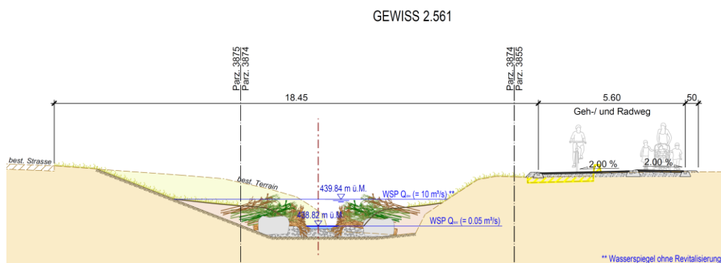
Abb. 54: Vorprojekt Profil Altbach/Veloweg (vbg, 2020)
