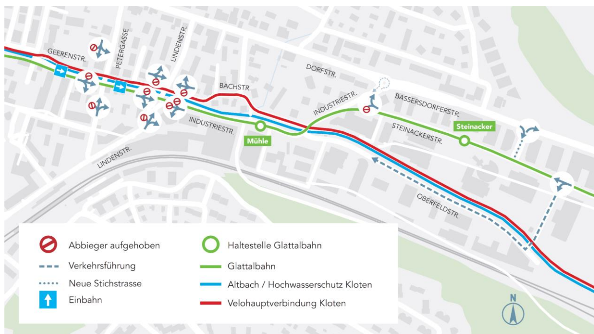
Abb. 48: Anpassung Verkehrsregime (VBG, 2020)
