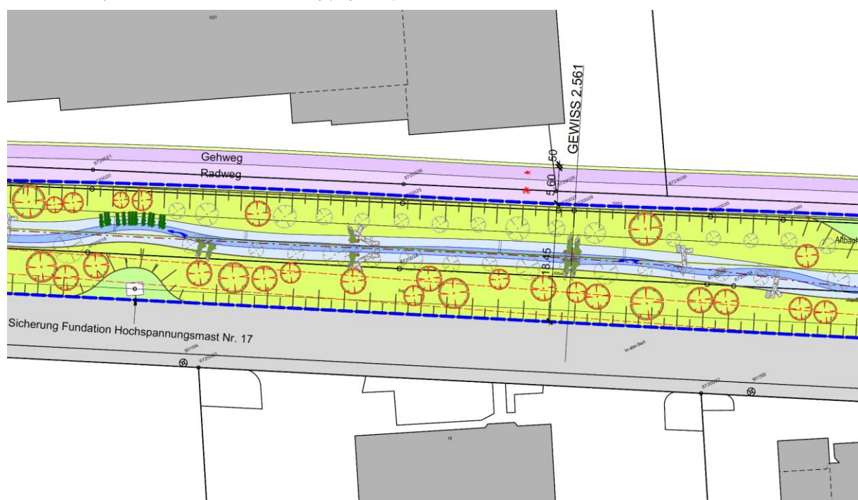
Abb. 55: Vorprojekt Situationsplan Altbach/Veloweg (vbg, 2020)
