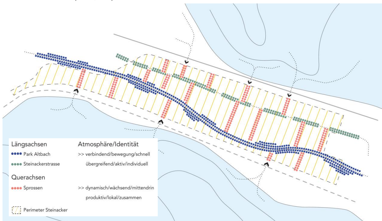
Abb. 33: Freiraumstruktur (LINEA, 2021)
